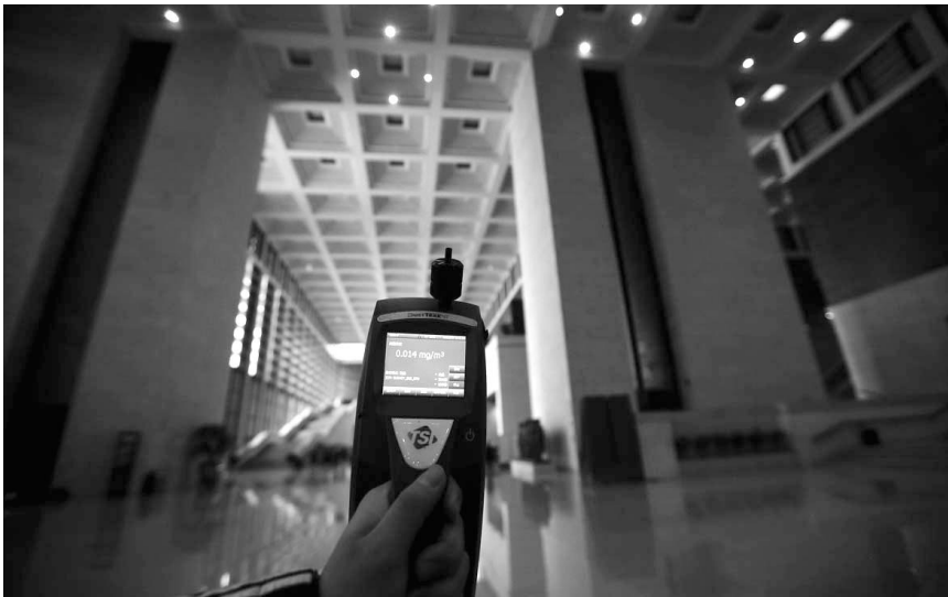
国家博物馆设置了20个环境监测点,每日派工作人员检测两次,并将检测数据输入电脑系统,确保空气质量。图为检测仪器显示PM2.5质量浓度为0.014mg/m³。
