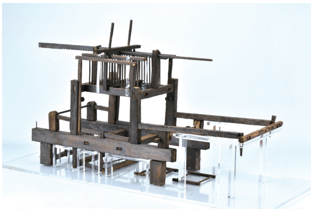
▲从左至右为滑框型一勾多综提花木织机模型和调丝木俑、纬络木俑 成都博物馆藏
